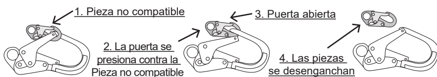
FIGURA 2: DESENGANCHE ACCIDENTAL
