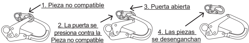
FIGURA 2: DESENGANCHE ACCIDENTAL
