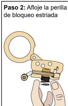
FIGURA 9 - INSTALACIÓN Y FUNCIONAMIENTO DEL AGARRADOR DE CUERDA DE EXTREMO LIBRE
