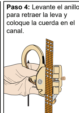
FIGURA 9 - INSTALACIÓN Y FUNCIONAMIENTO DEL AGARRADOR DE CUERDA DE EXTREMO LIBRE
