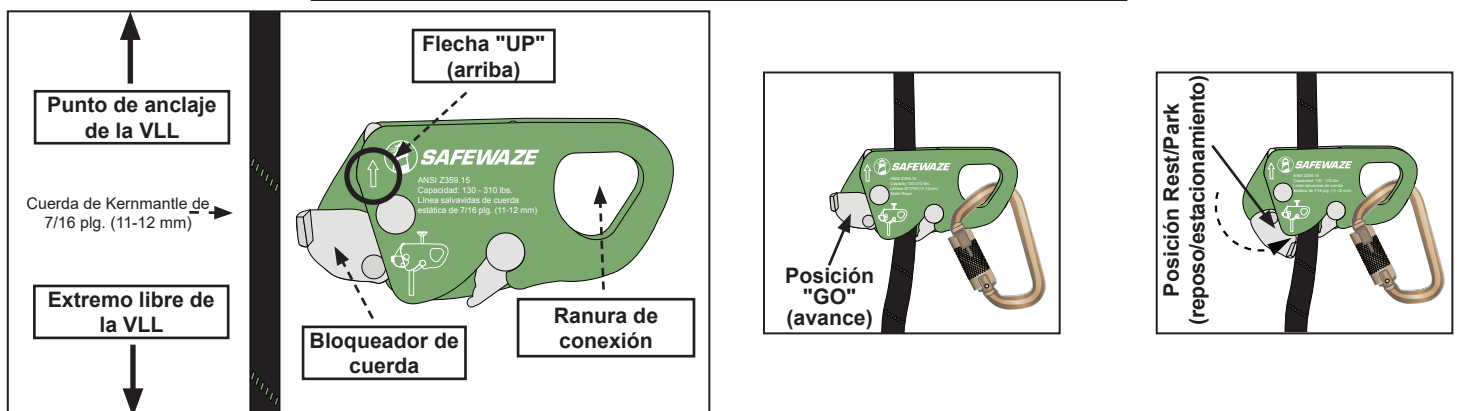
FIGURA 12 - INSTALACIÓN
