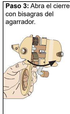
FIGURA 9 - INSTALACIÓN Y FUNCIONAMIENTO DEL AGARRADOR DE CUERDA DE EXTREMO LIBRE
