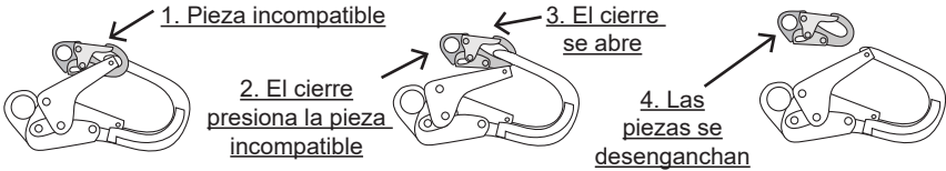
FIGURA 2: DESENGANCHE NO INTENCIONAL
