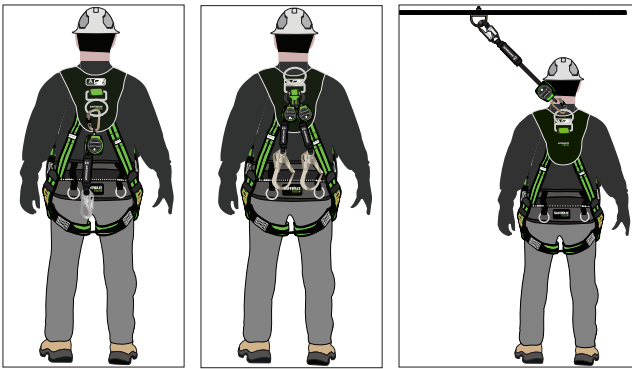
FIGURA 4: EJEMPLOS DE CONEXIÓN
