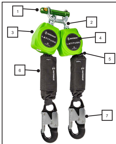
IMÁGENES 4 y 5: INSPECCIÓN DE UNIDADES DE CORREA TEJIDA LATITUDE
