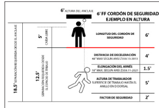
FIGURA 1: Diagrama de Espacio Libre para Caídas
