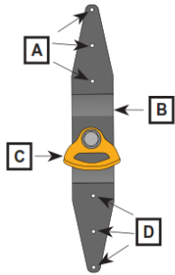
FIGURA 5 - COMPONENTES DEL ANCLA
