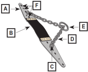
FIGURA 5 - COMPONENTES DEL ANCLA DE CADENA
